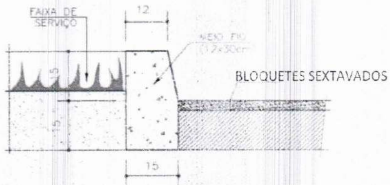
CORTE ESQUEMÁTICO DO MEIO FIO
