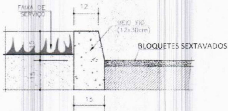
CORTE ESQUEMATICO DO MEIO FIO
