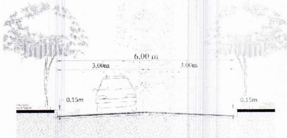
SEÇÃO TIPO DE PAVIMENTAÇÃO
