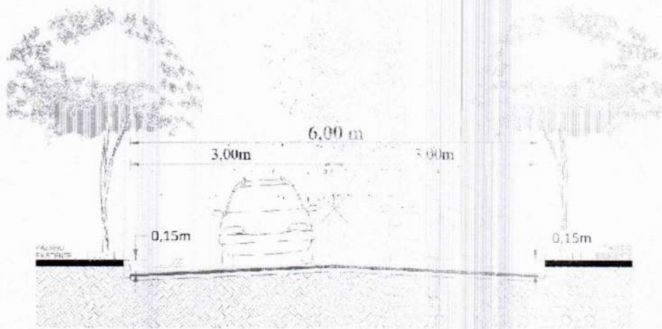
SEÇÃO TIPO DE PAVIMENTAÇÃO
