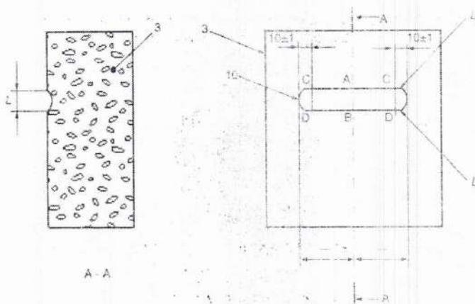
Figura C.2 — Medição da cavidade na amostra ensaiada
