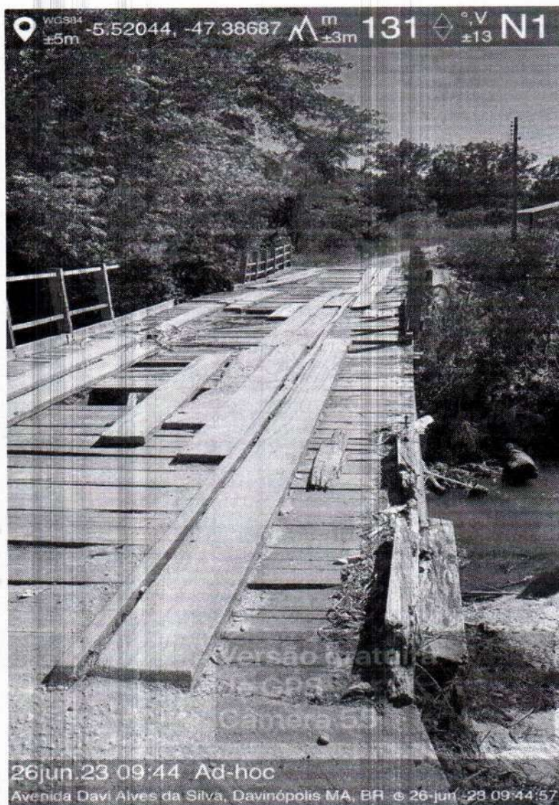
Foto 02 – Rodeiro e Guarda-corpo destiorado.
