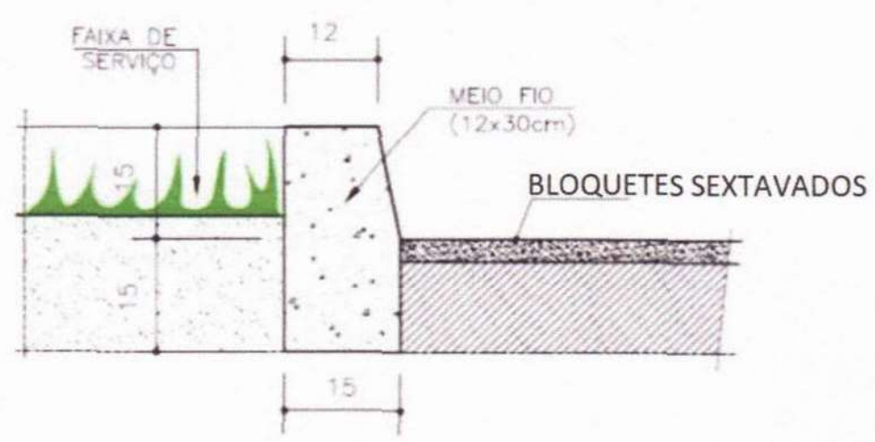
CORTE ESQUEMÁTICO DO MEIO FIO
