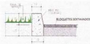
CORTE ESQUEMÁTICO DO MEIO FIO
