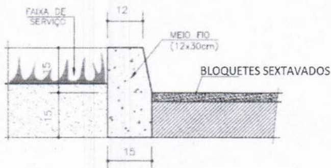
CORTE ESQUEMÁTICO DO MEIO FIO
