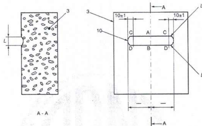
Figura C.2 — Medição da cavidade na amostra ensaiada
