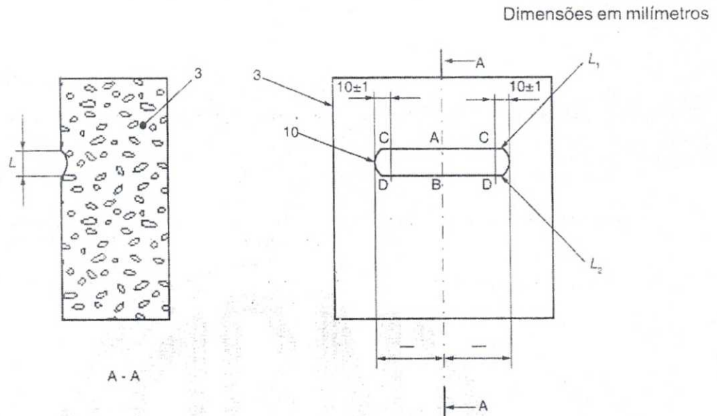
Figura C.2 — Medição da cavidade na amostra ensaiada
